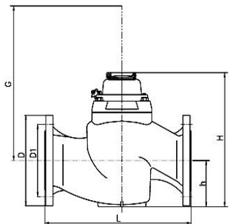
垂直螺翼式水表
