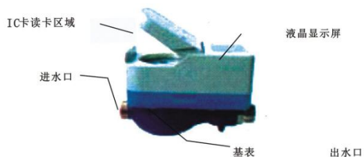
图 2 水表外观
