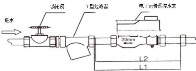
安装示意图
